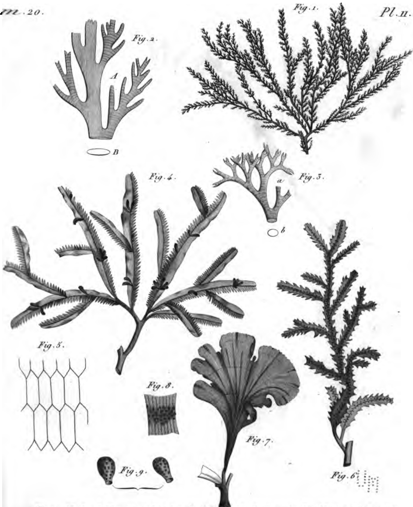
Fig. 1. 2. AB 3 a b, Plocamium Cristatum. Fig. 4, 5 Amansia Semipennata. Fig. 6 Dictyopteris Serrulata.
